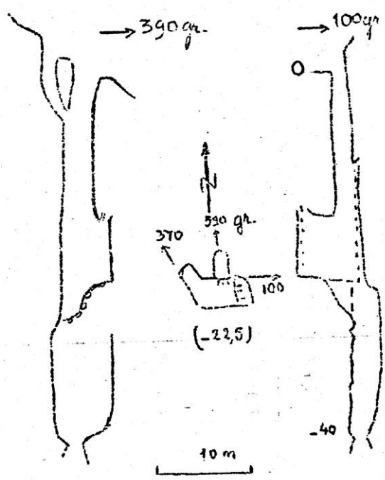
Plan, coupes 505
